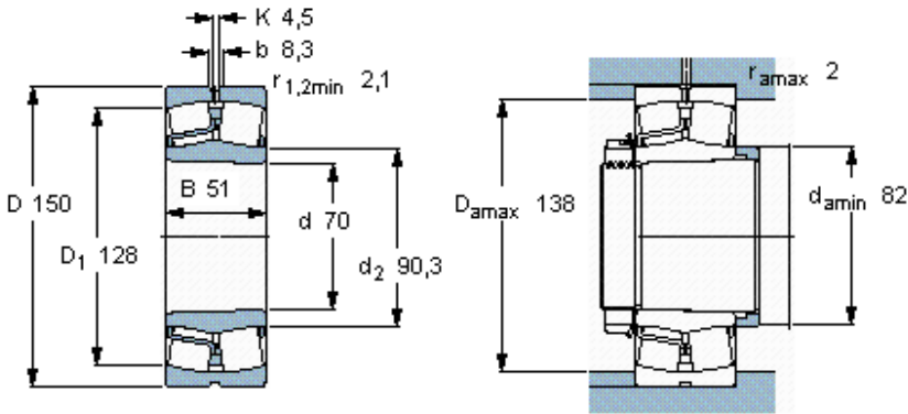
Kuželová díra, kuželovitost 1: 12
